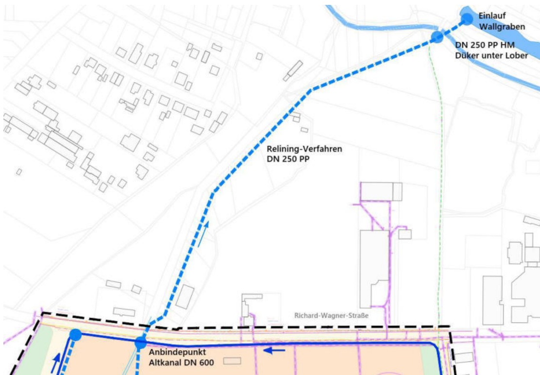
Abbildung 24: Trassenverlauf äußere Erschließung
