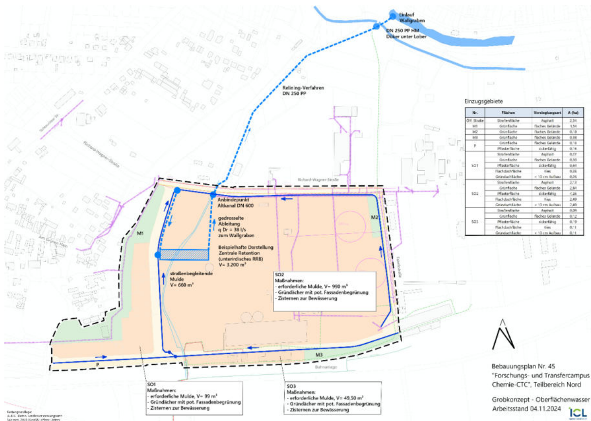
Abbildung 45: Grobkonzept Oberflächenwasser; Auszug aus dem Gesamtentwässerungskonzept © ICL 2024
