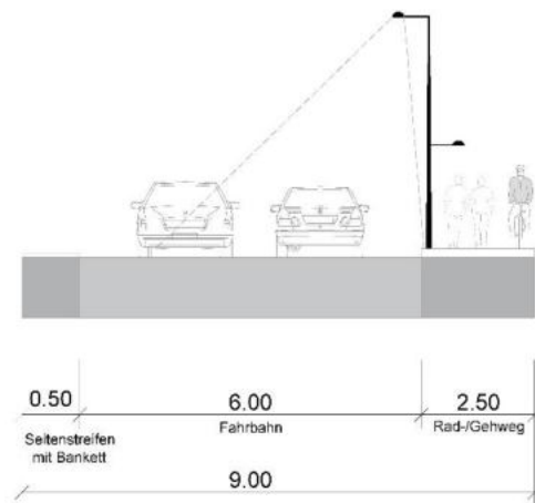
Abbildung 42: Regelquerschnitt Planstraße B (keine Festsetzung) © ICL
