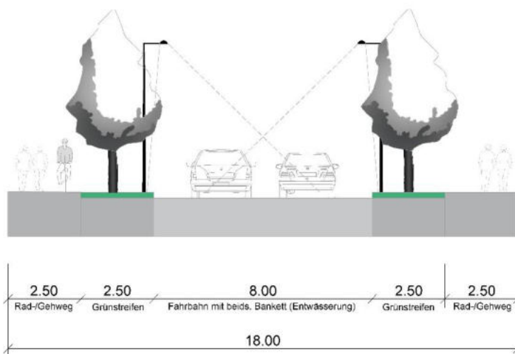
Abbildung 39: Regelquerschnitt Planstraße A, keine Festsetzung © ICL
